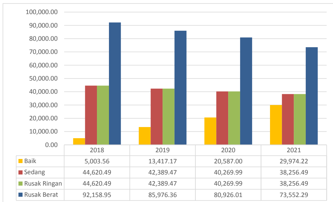
Gambar 2.31. Panjang Drainase Sistem Terbuka Berdasarkan Kondisi di Kota Jambi Tahun 2018-2021
