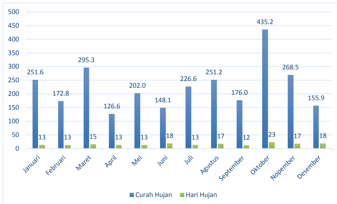
Gambar 2.6. Curah Hujan dan Hari Hujan Menurut Bulan Tahun 2022
