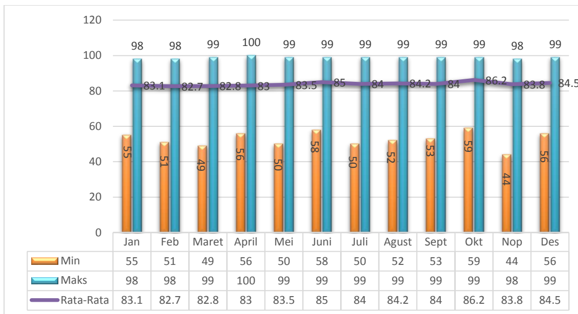
Gambar 2.5. Kelembaban Udara Minimum, Maksimum dan Rata-Rata Menurut Bulan Tahun 2022
