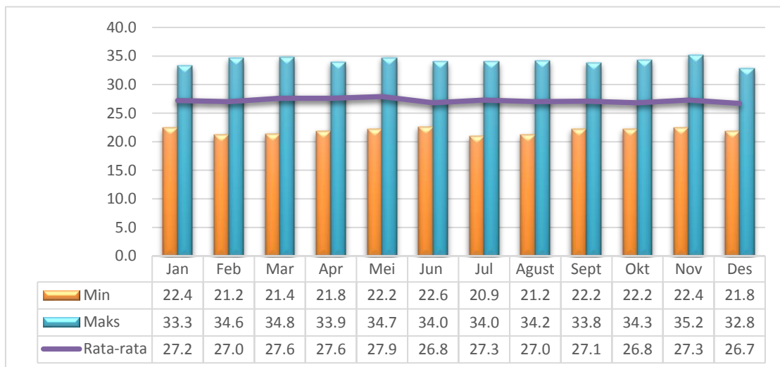
Gambar 2.4. Suhu/Temperatur Minimum, Maksimum dan Rata-Rata Menurut Bulan Tahun 2022
