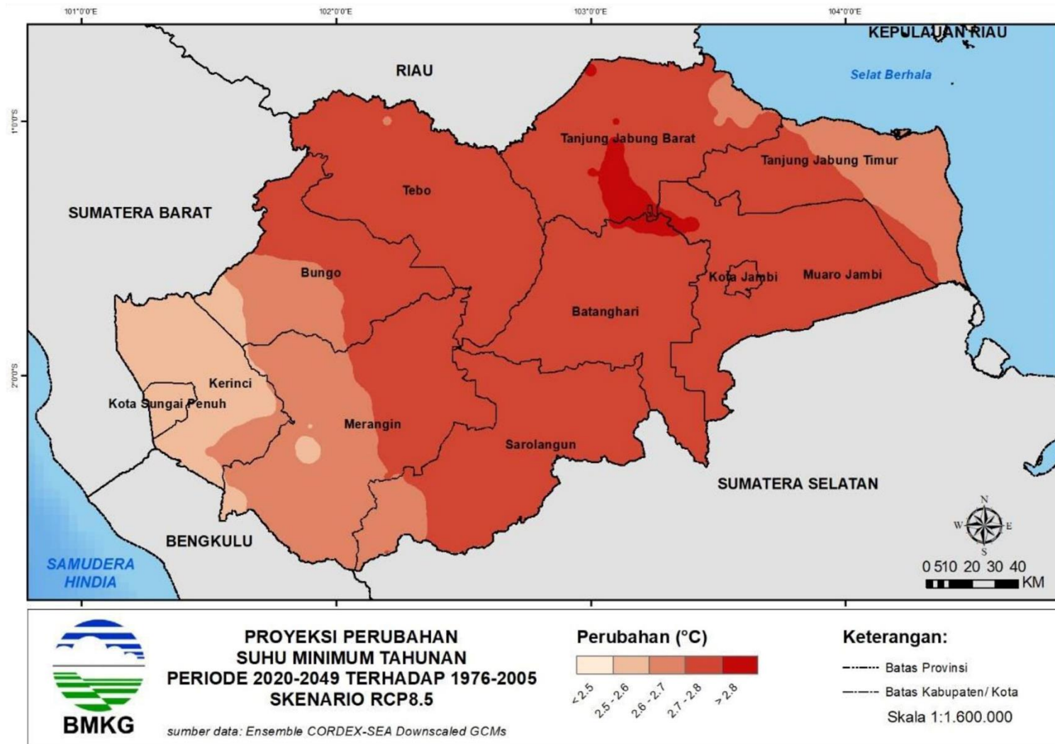
Gambar 8. Proyeksi temperatur minimum
