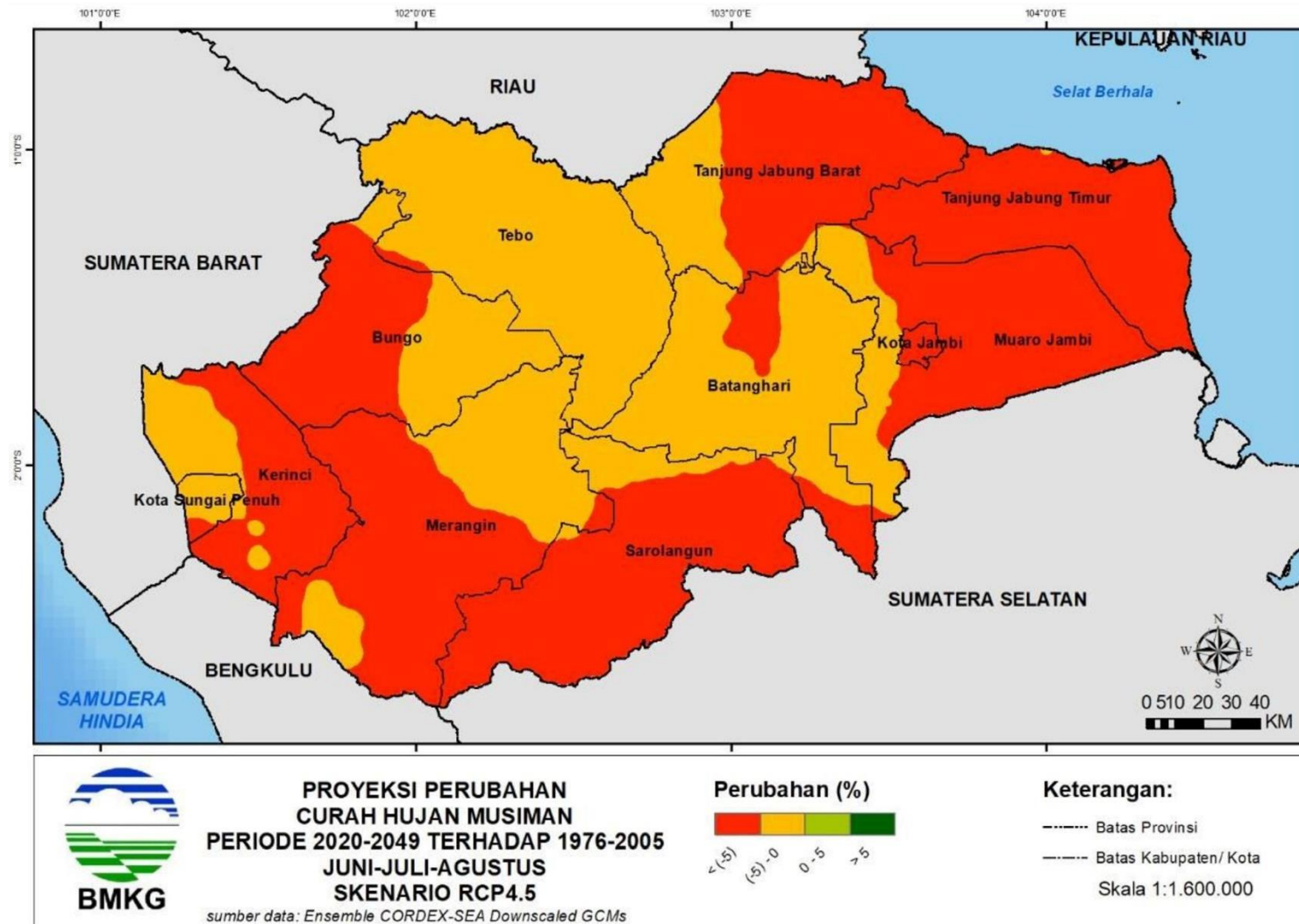
Gambar 11. Proyeksi hujan JJA (Juni-Juli-Agustus)
