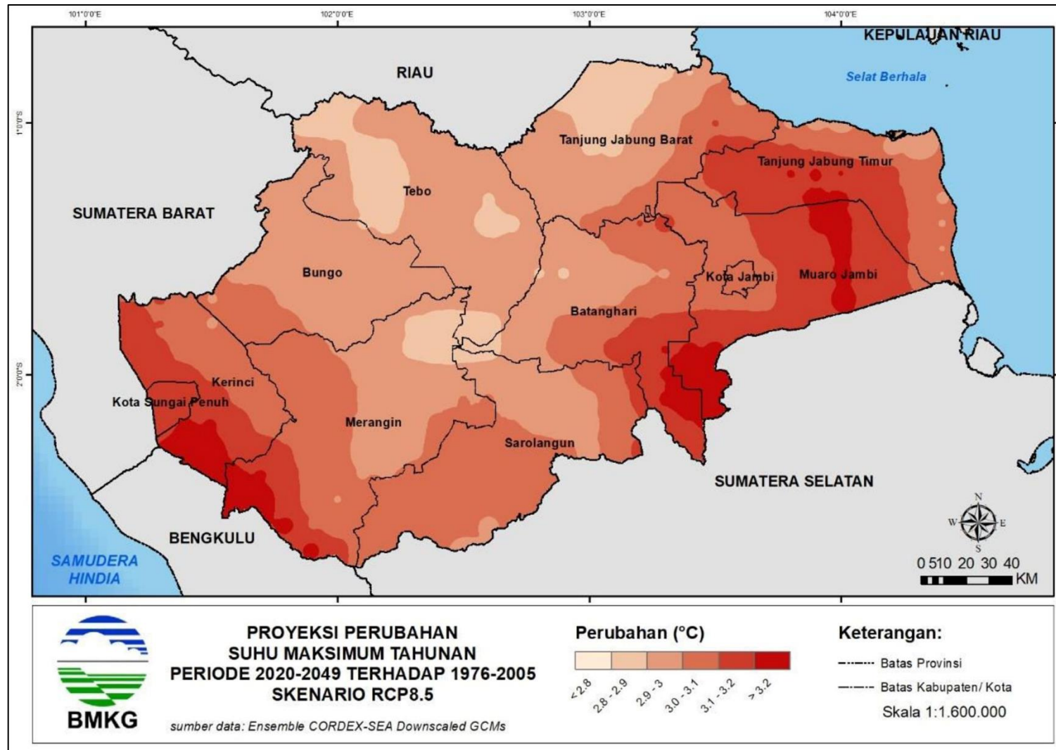
Gambar 7. Proyeksi temperatur maksimum
