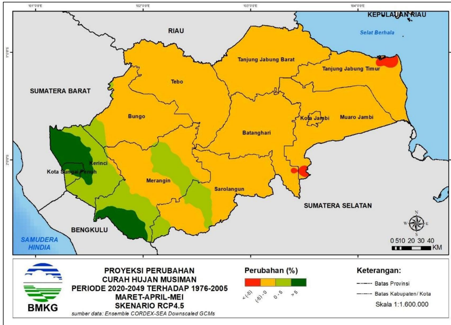
Gambar 10. Proyeksi hujan MAM (Maret-April-Mei)
