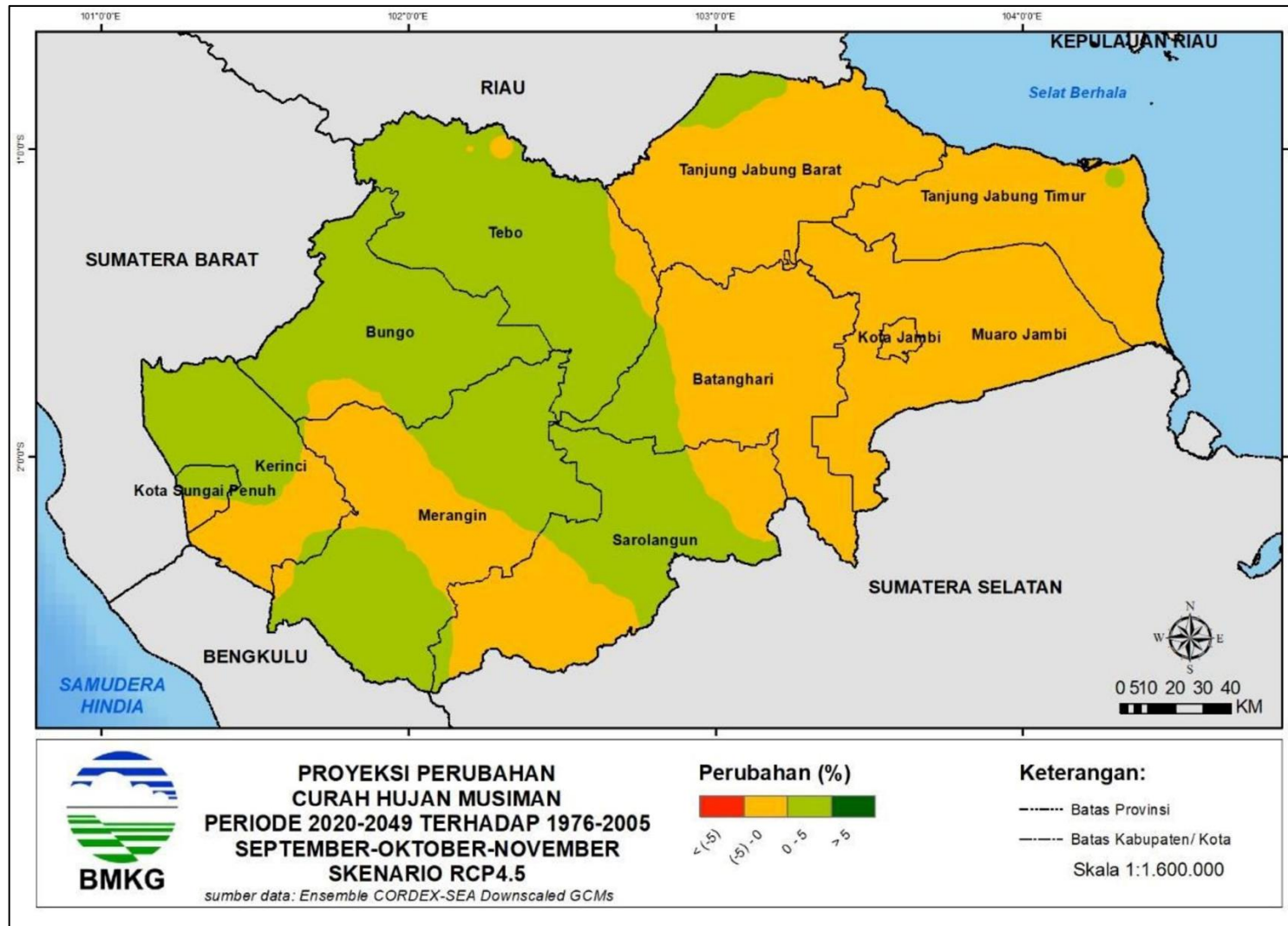
Gambar 12. Proyeksi hujan SON (September-Oktober-November)
