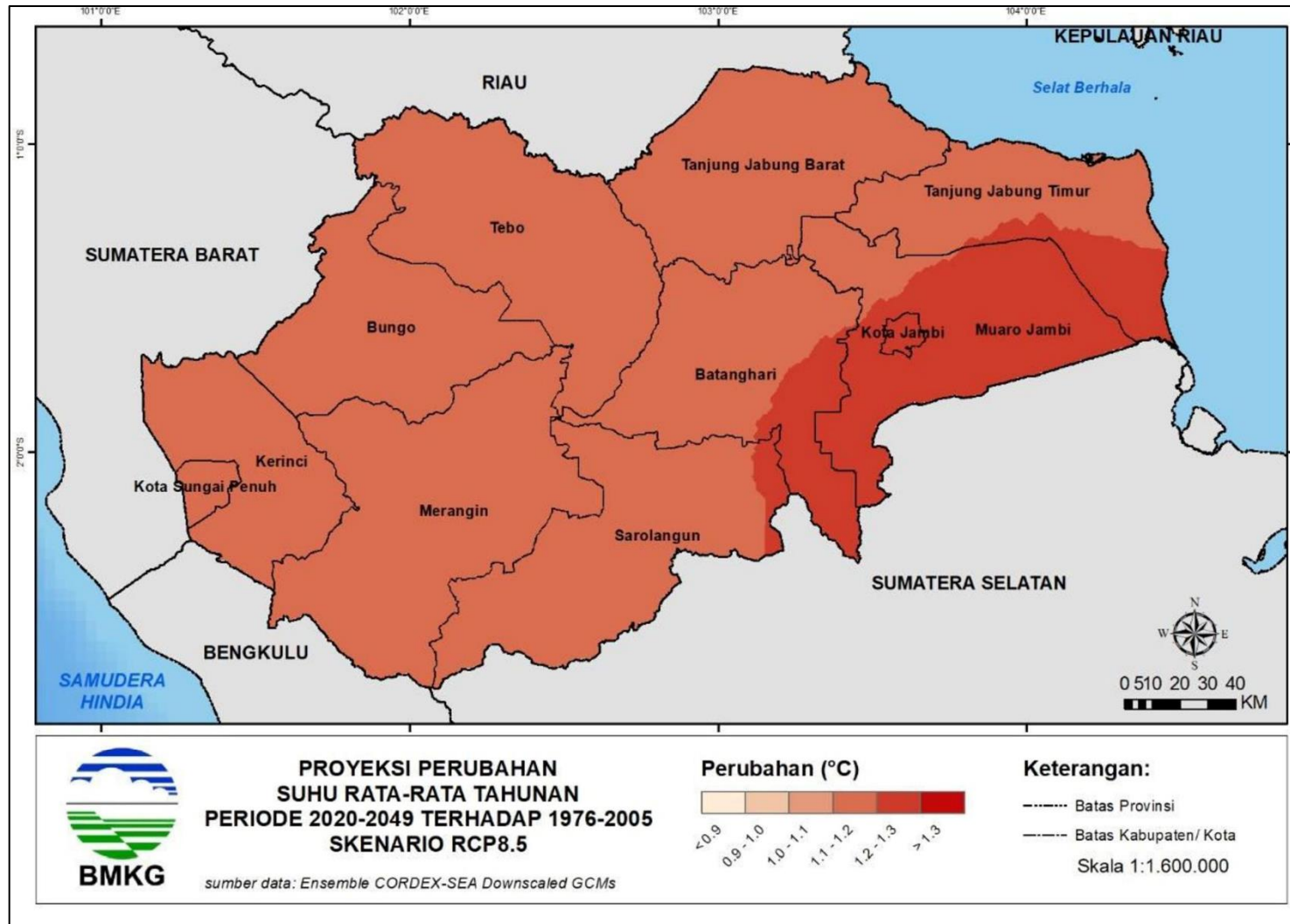
Gambar 6. Proyeksi temperatur rata-rata
